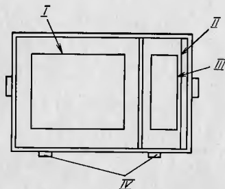
Рис.45. Схема размещения прибора и комплекта ЭИП в укладочном ящике: I - прибор; II - эксплуатационная документация; III - комплект ЭИП; IV - места пломбирования
