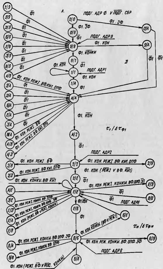
Рис. 11. - Диаграмма состояний блока I-K триггеров
