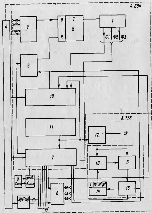
Рис.10. Схема электрическая структурная делителя:
