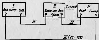
Рис.36. Схема соединений генератора Г5-79 с осциллографом СИ-108 при измерении малых временных сдвигов: I - поверяемый генератор Г5-60; II - испытываемый генератор Г5-79; III - осциллограф СИ-108; IV - кабель В4
