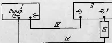
Рис.25. Схема соединений генератора Г5-79 с осциллографом СИ-108 при работе с амплитудой сигналов до 9,9 В: I - поверяемый генератор Г5-79; II - осциллограф СИ-108; III - переход 32-ИЛ4/3; IV - кабель ВЧ (комплект СИ-108)
