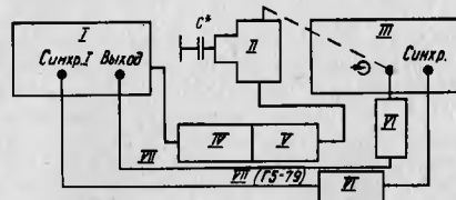
Рис.30. Схема соединения приборов для определения погрешности установки амплитуды на выходе 1 кОм (выносной блок) с помощью осциллографа С1-65А:
