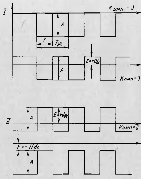
Рис.16. Подключение базового смещения E к выходному сигналу: I - неинвертируемые сигналы; II - инвертируемые сигналы
