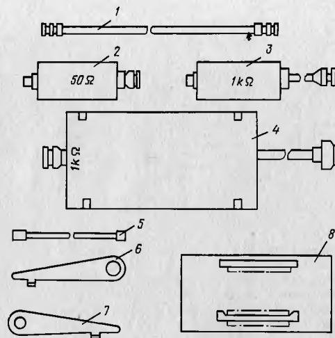
Рис.2. Основные принадлежности комплекта ЗИП:
