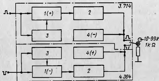
Рис.18. Схема электрическая функциональная блока выносного: 1 - усилитель; 2 - эмиттерный повторитель; 3 - формирователь среза ("top"); 4 - дополнительный источник тока
