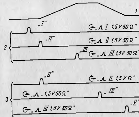
Рис.35. Временные диаграммы:
