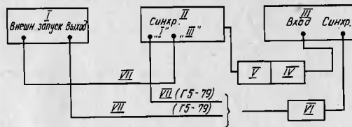
Рис.41. Схема соединений поверяемого генератора с осциллографом СИ-65А для определения длительности фронта и среза: I - генератор импульсов Г5-60; II - поверяемый генератор Г5-79; III - осциллограф СИ-65А; IV - нагрузка I кОм; V - выносной блок; VI - нагрузка 50 Ом; VII - кабель ВЧ
