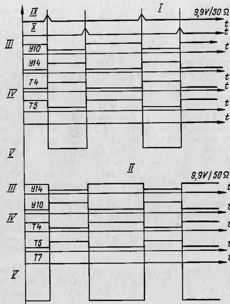
Рис.15. Временные диаграммы:
