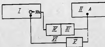
Рис.39. Схема соединений поверяемого генератора с частотомером ЧЗ-54 при определении количества импульсов в серии: I - поверяемый генератор Г5-79; II - частотомер ЧЗ-54; III - нагрузка I кОм; IV - выносной блок; V - нагрузка 50 Ом; VI - кабель ВЧ (Г5-79)
