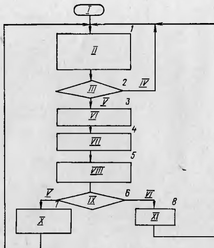
Рис.6. Алгоритм управляющей программы:
