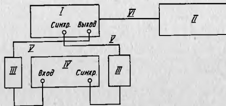
Рис. 26. Схема соединений испытываемого генератора Г5-79 с анализатором логических состояний:
