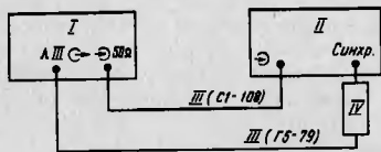
Рис.32. Схема соединений поверяемого генератора с осциллографом СИ-108 при определении малых длительностей: I - генератор Г5-79; II - осциллограф СИ-108; III - кабель ВЧ; IV - переход 0.364.030
