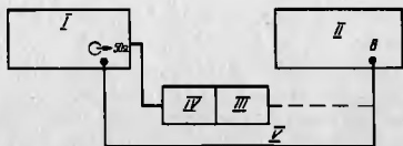
Рис.31. Схема соединений поверяемого генератора с частотомером ЧЗ-54 при определении длительности импульсов: I - генератор Г5-79; II - частотомер ЧЗ-54; III - нагрузка I кОм; IV - выносной блок; V - кабель ВЧ (Г5-79)
