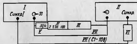
Рис.29. Схема соединения приборов для определения погрешности установки амплитуды на выходе 50 Ом с помощью осциллографа С1-108:
