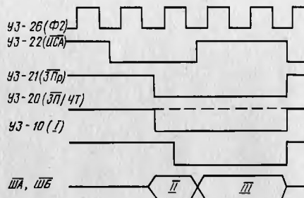
Рис.5. Временная диаграмма работы ОМП с ВП: I - ответ; II - адрес ВП; III - информация ОМП \Rightarrow ВП
