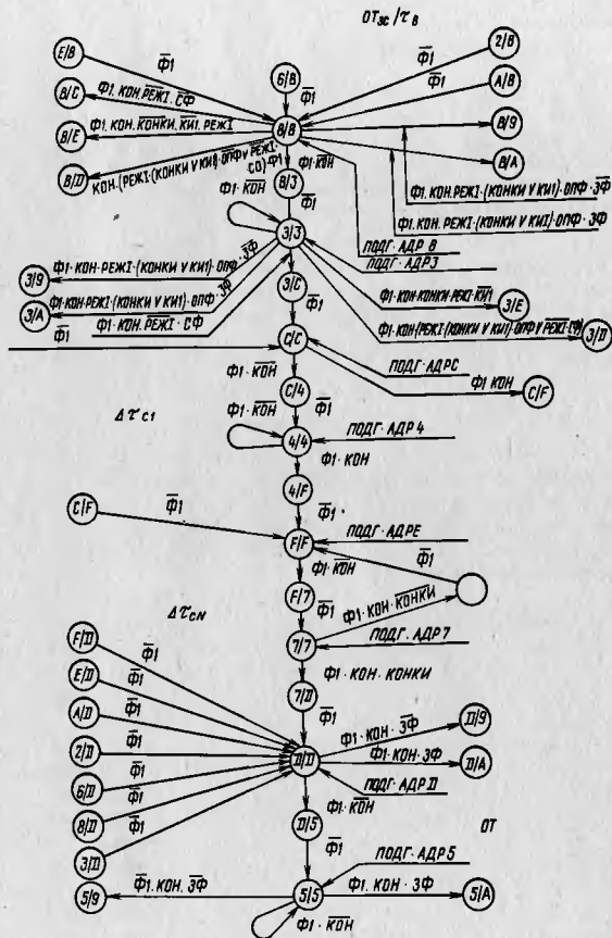
Рис. 12. Диаграмма состояний блока I-K триггеров
