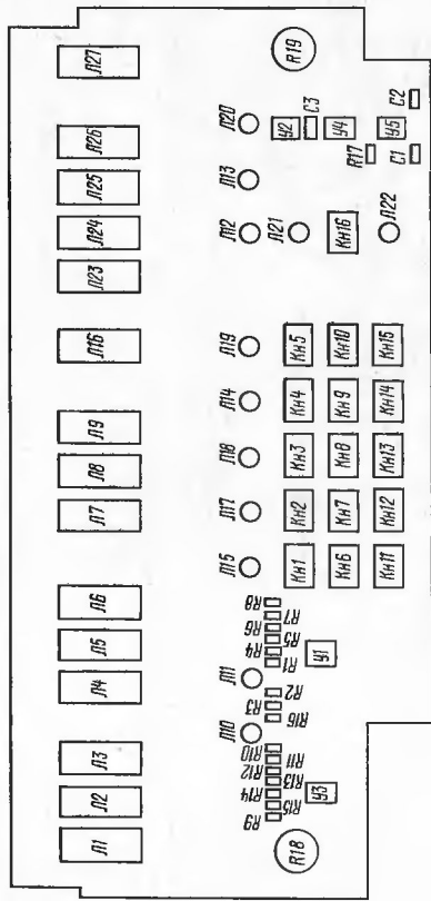
Рис. 4. Плата устройства цифровой индикации 3.644.
