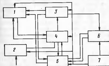
Рис.3. Электрическая функциональная схема генератора И5-75: 1 - блок цифровой индикации; 2 - линия коллективного пользования; 3 - делитель; 4 - устройство управления; 5 - цифроаналоговый преобразователь; 6 - блок выносной; 7 - стабилизатор
