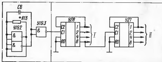
Рис.5. Схема электрическая функциональная генератора и адресных счетчиков: I - номер микротакта; II - номер такта
