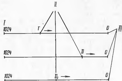
Рис.20. Диаграмма работы реверсивных счетчиков в режиме вычитания: I - числа в двоичном коде; II - запись установленных чисел; III - импульсы на выходе "обратный перенос" счетчика при вычитании Пример: T=574 ; D=223 ; D_1 = D + \tau \approx 223 + 271 = 494
