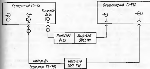
Рис.33. Схема электрическая соединения генератора Г5-75 с осциллографом С1-65А
