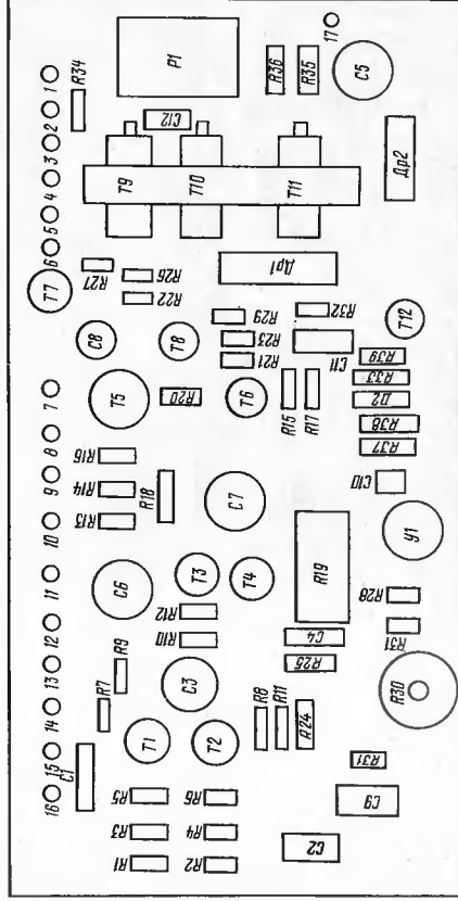
Рис.6. Плата формирователя 3.636
