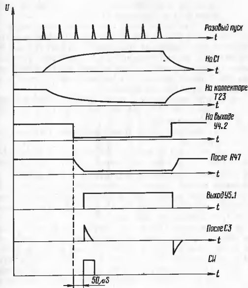
Рис.24. Временная диаграмма работы схемы формирования синхроимпульсов
