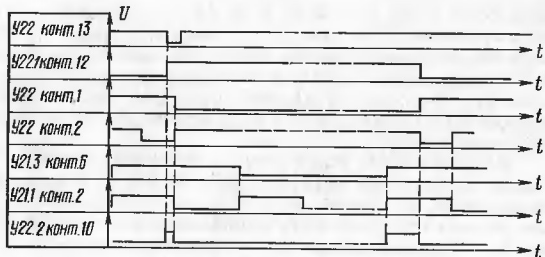
Рис.10. Диаграмма работы схемы разрешения записи
