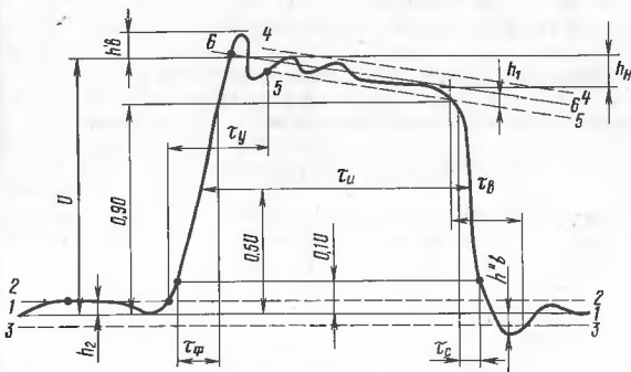
Рис.41. Усредненная форма основного импульса генератора: 1-1 - исходный уровень; 2-2, 3-3 - пределы допускаемой неравномерности в паузе; 4-4, 5-5 - пределы допускаемой неравномерности вершины; 6-6 - усредненная вершина импульса; U - амплитуда импульса; \tau_u - длительность импульса; \tau_f , \tau_c - длительность фронта, среза; h' , h , h' - выбросы на вершине и в паузе; h_1 , h_2 - неравномерность вершины и в паузе; h_n - наклон вершины (часть неравномерности вершины); \tau_u , \tau_b - время установления и восстановления
