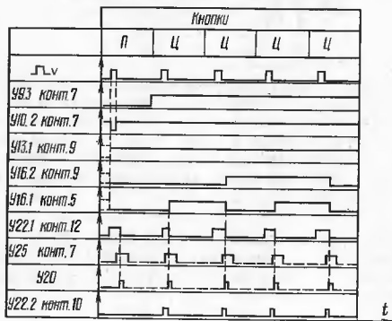
Рис. 9. Диаграмма работы схемы записи в память по алгоритму П-Ц-Ц
