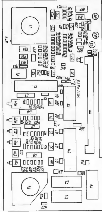
Рис. 8. Панель стабилизатора напряжения 3.638
