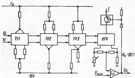
Рис.26. Схема электрическая функциональная формирователя выходных импульсов положительной полярности: ТК1 – ТК3 – токовый ключ; БТК – выходной токовый ключ; U_K – калибровочное напряжение
