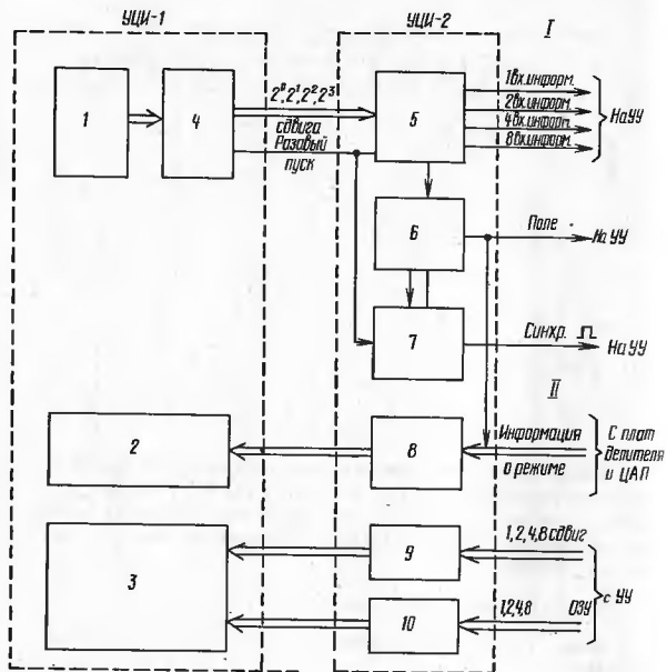
Рис.23. Схема электрическая функциональная блока цифровой индикации: I - кнопочное поле; 2 - лампы индикации режимов; 3 - лампы индикации информации; 4 - охема опроса кнопок; 5 - схема получения и хранения кода кнопки; 6 - схема формирования сигнала "поле"; 7 - охема формирования синхроимпульса; 8 - инверторы; 9 - схема выбора ламп; 10 - схема выбора сегментов I - выходные сигналы; II - входные сигналы
