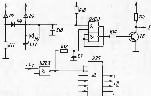
Рис. 6. Схема электрическая принципиальная выбора номера программы: I - на вход ОЗУ; II - адрес столбца ОЗУ; III - память
