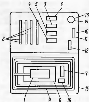
Рис.2. Комплект ЗИП: 1 - выносной блок; 2 - аттенуатор *20 дБ; 3 - нагрузка *50 \Omega 1W; 4 - нагрузка *50 \Omega 2W; 5 - аттенуатор *40 дБ; 6 - плата; 7 - кабель 4.853.22I; 8 - кабель 4.853.222; 9 - кабель соединительный В4; 10 - рычаг 8.332.057; 11 - рычаг 8.332.057-01; 12 - индикатор вакуумный люминесцентный ИВ-8; 13 - лампа СМН 6,3-20-2; 14 - вставка плавкая ВП-I-IА; 15 - укладочный ящик; 16 - тройник 3.649.000
