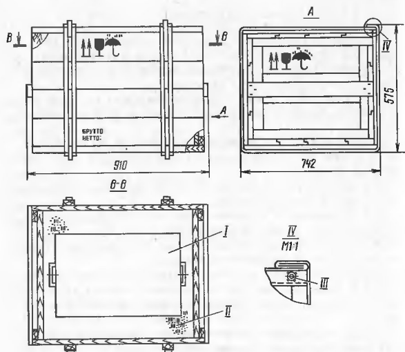
Рис. 42. Транспортный ящик. Маркировка и места расположения пломб: I - изделие в укладочном ящике; II - упаковочный материал; III - пломба
