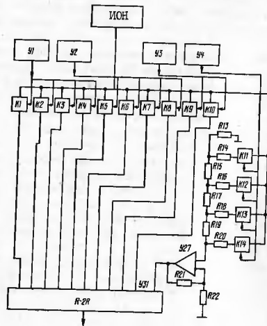
Рис.16. Схема электрическая функциональная ЦАП
