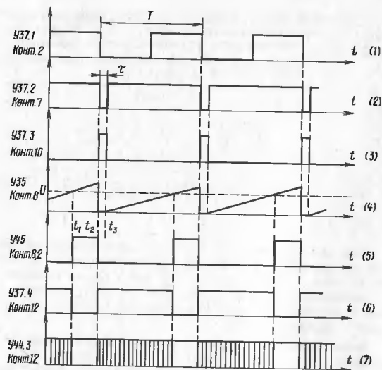
Рис.17. Диаграмма работы АЦП
