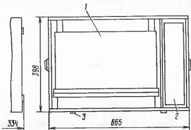
Рис. 43. Размещение генератора и ЗИП в укладочном ящике (вид без крышки): I - генератор; 2 - комплект ЗИП; 3 - место пломбирования
