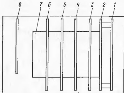
Рис.31. Карта расположения плат в основном блоке в приборе (вид сверху)
