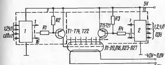
рис. 25. Схема электрическая функциональная управления сетками и сегментами индикаторных ламп: 1 - дешифратор ламп, 2 - дешифратор сегментов
