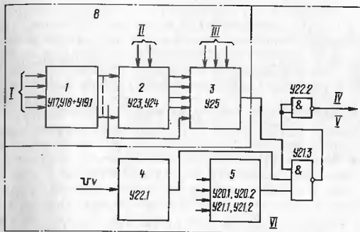
Рис. 7. Схема электрическая функциональная формирователя импульса записи в ОЗУ: I - дешифратор; 2 - мультиплексор разряда; 3 - мультиплексор параметра; 4 - RS - триггер; 5 - схема формирования запрета записи; I - номер такта; II - номер разряда; III - номер параметра; IV - на вход ОЗУ; V - запись (считывания); VI - запрет записи на время первого микротакта
