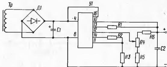
Рис.28. Схема электрическая принципиальная включения стабилизатора напряжения на микросхеме
