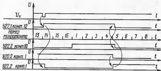
Рис. 8. Диаграмма работы RS - триггера
