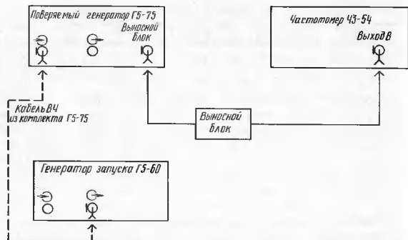
Рис.39. Схема электрическая соединения приборов при определении длительности импульсов
