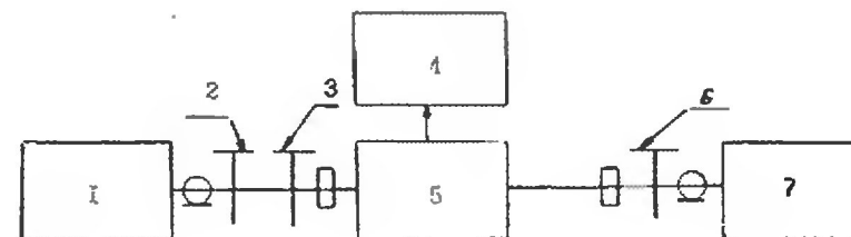
Рис. 7. Схема электрическая структурная для измерения K_{сг} преобразователя с переходом 2.236.016 на входе из частоте 12 ГГц.
