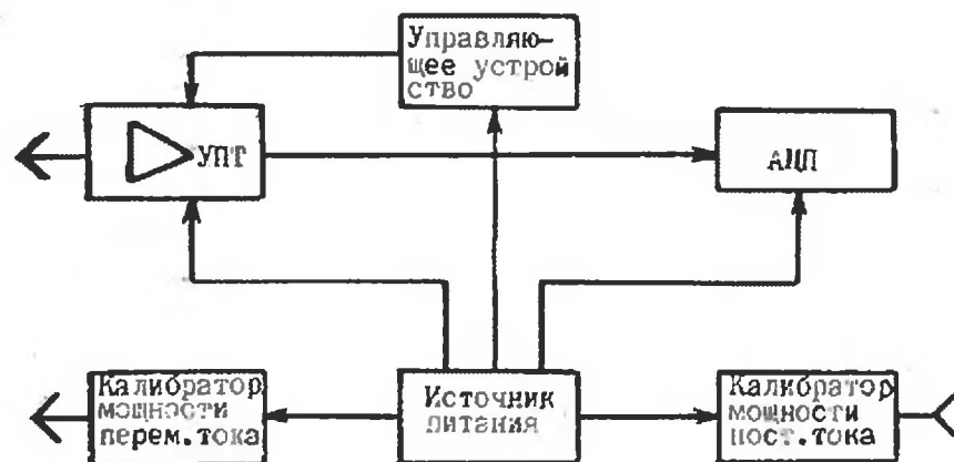
Рис. 2. Схема электрическая структурная измерительного блока ваттметра
