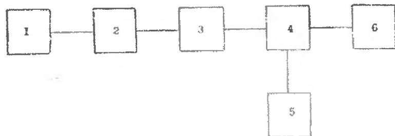
Рис. 5. Схема электрическая структурная для проверки Кет и измерительного преобразователя в диапазоне частот 3—17,85 ГГц
