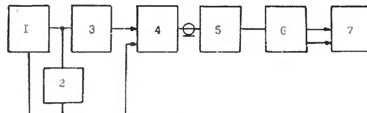
Рис. 8. Схема электрическая структурная для измерения коэффициента преобразования измерительных преобразователей на постоянном токе.
