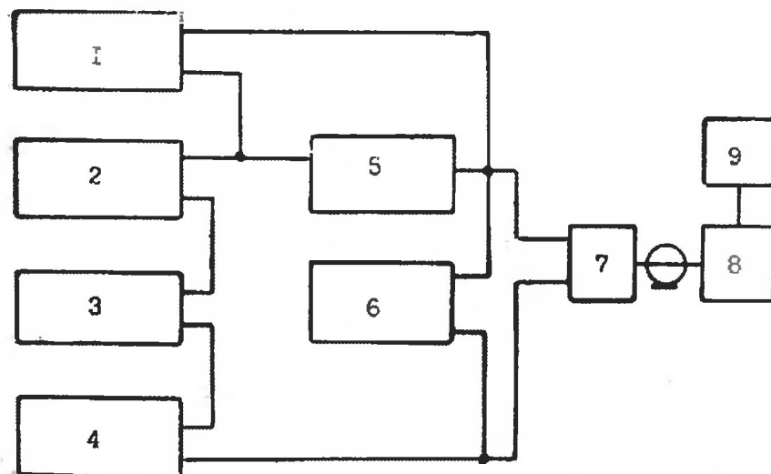
Рис. 9. Схема электрическая структурная для измерения нелинейности ваттметра
