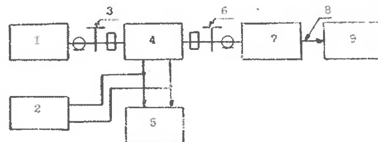
Рис. 6. Схема электрическая структурная для измерения коэффициента эффективности измерительного преобразователя на частоте 12 ГГц
