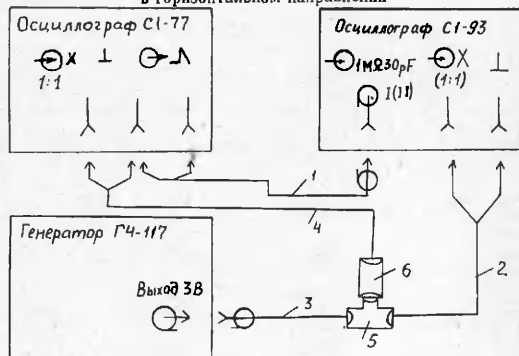
Структурная схема измерения ширины линии луча в горизонтальном направлении
