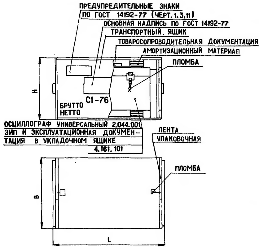
Схема упаковки и маркирования упаковки
