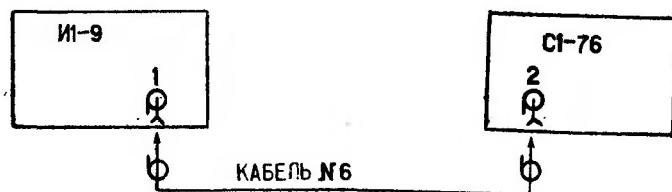
Схема соединения приборов для определения погрешности коэффициента отклонения
