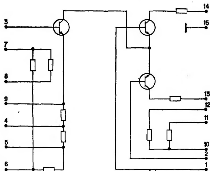
Микросхема Усилитель регулируемый 228УВ2
