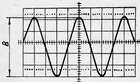
Рис. 12. Принцип измерения размаха напряжения
