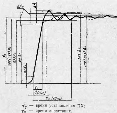
Рис. 17. Измерение времени нарастания, выброса, неравномерности вершины на участке установления ПХ
