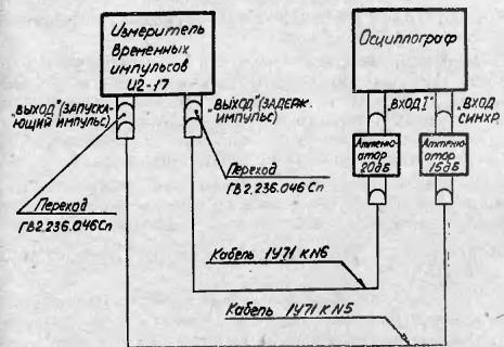
Рис. 32. Схема соединения приборов для определения погрешности коэффициентов развертки осциллографа с блоком Я40-2700 (1Р71)
