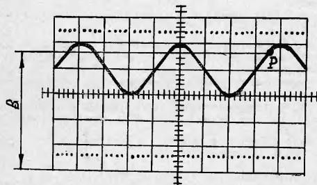
Рис. 13. Принцип измерения мгновенного значения напряжения
