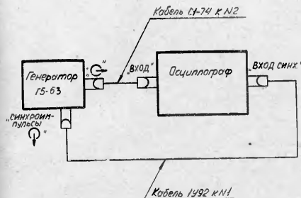
Рис. 24. Схема соединения приборов для определения времени нарастания ПХ осциллографа с блоком Я40-1901 (1У92)
