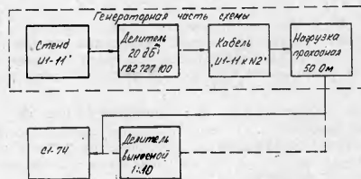
Рис. 22. Схема соединения приборов при проверке времени нарастания, величины выброса и времени установления ПХ осциллографа с блоком Я40-1900 (1У91)
