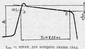
Рис. 17а. Определение спада ПХ
