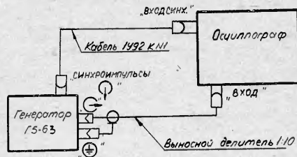
Рис. 26. Схема соединения приборов для определения времени нарастания ПХ осциллографа с блоком Я40-1901 (1932) и выносным делителем 1:10
