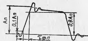
Рис. 8. Изображение импульса на экране ЭЛТ при измерении времени нарастания переходной характеристики
