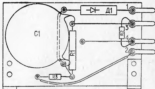
Рис. 11. Маркировочная схема высоковольтного усилителя.
