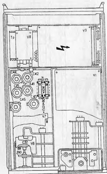
Рис. 3. Схема расположения установочных элементов и печатных плат (вид снизу)
