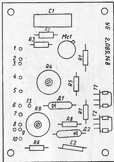
Рис. 7. Маркировочная схема калибратора амплитуды и длительности.
