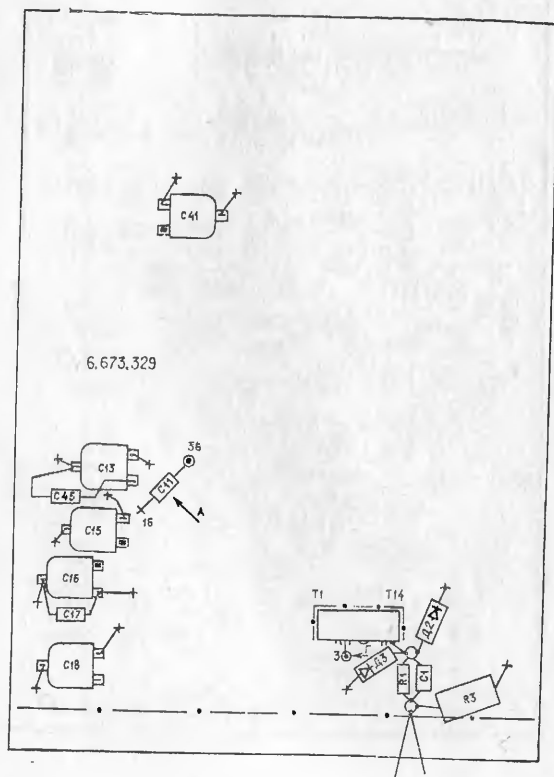
Рис. 2. Маркировочная схема предусилителя вертикального отклонения и синхронизации (оборотная сторона платы).
