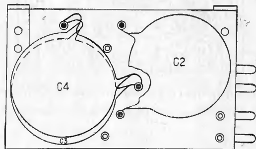
Рис. 12. Маркировочная схема высоковольтного усилителя (оборотная сторона).
