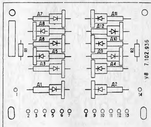
Рис. 9. Маркировочная схема выпрямителя стабилизатора +10, -10, +80 и 150 В
