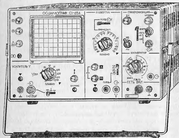
Рис. 1. Общий вид осциллографа
