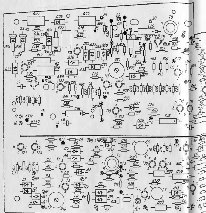
Рис. 5. Маркировочная схема блока развертки, сдвига и усилителя горизонтального отклонения.
