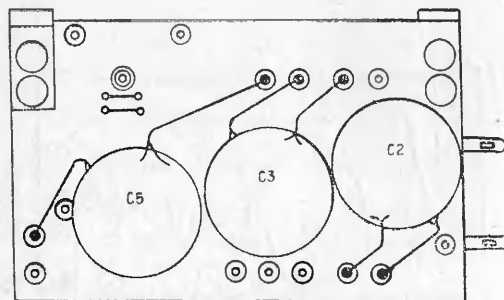
Рис. 13. Маркировочная схема выпрямителя высоковольтного.
