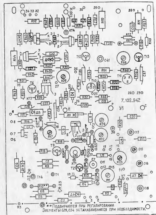
Рис. 1. Маркировочная схема предусилителя вертикального отклонения и синхронизации.
