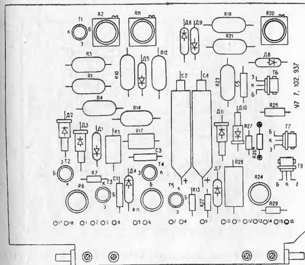
Рис. 8. Маркировочная схема блока питания.
