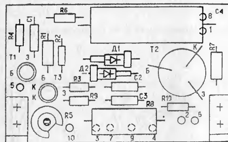
Рис. 10. Маркировочная схема платы высоковольтного преобразователя.
