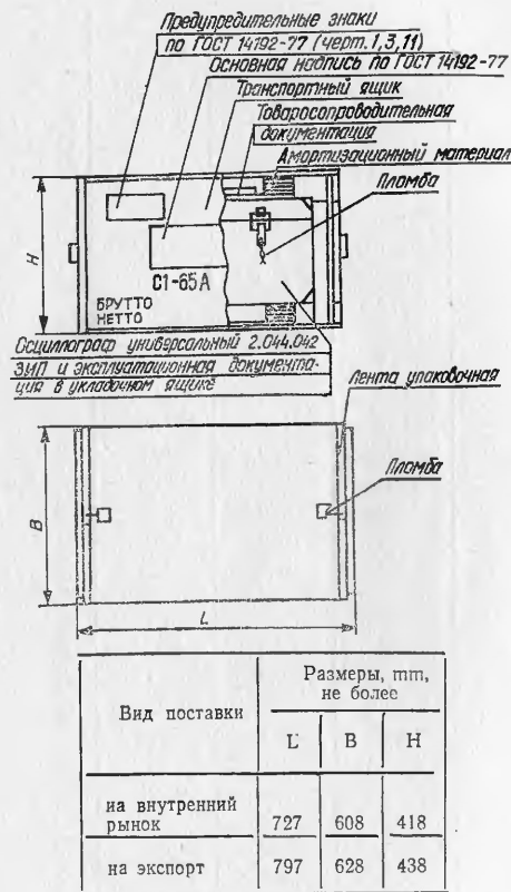
Рис. 11. Схема упаковки и маркирования упаковки
