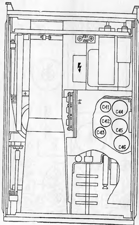
Рис. 2. Схема расположения установочных элементов и печатных плат (вид сверху).
