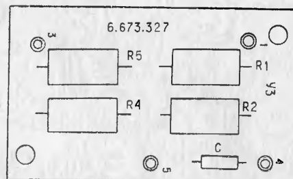
Рис. 4. Маркировочная схема электрических нагрузок.
