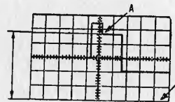
Рис. 4. Измерение мгновенного постоянного напряжения относительно контрольной линии
