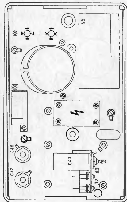
Рис. 5. Задняя стенка осциллографа. Расположение установочных элементов и печатных плат
