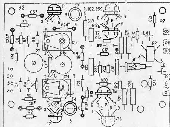
Рис. 3. Маркировочная схема выходного усилителя.
