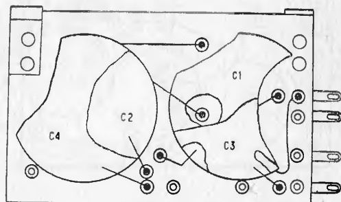
Рис. 14. Маркировочная схема выпрямителя высоковольтного 1,5 kV.
