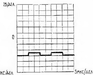
Рис. 24. База транзистора Т3
