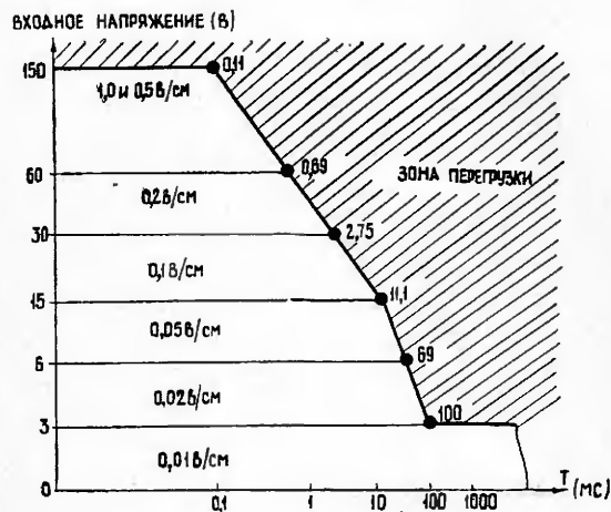
Рис. 15. Зависимость величины импульсного входного напряжения от длительности импульса T для сигналов со средней мощностью 0,25 Вт и частотой следования более одного в минуту
