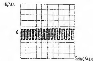
Рис. 6. Эмиттер транзистора Т23
