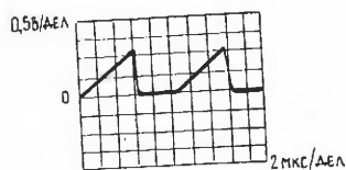
Рис. 16. Эмиттер транзистора T30
