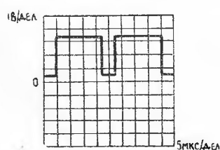
Рис. 3. Коллектор микросхемы МС1-2
