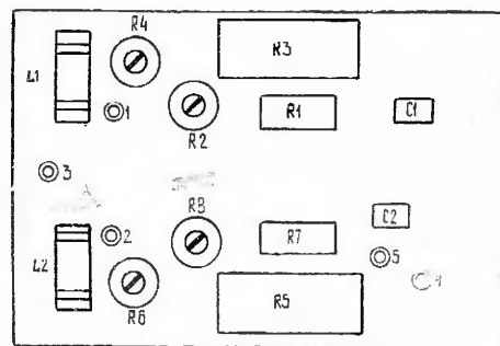
Рис. 11. Расположение элементов на плате управления
