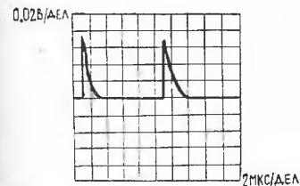
Рис. 31. База транзистора Т1
