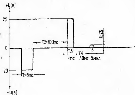
Рис. 16. Форма сложного импульсного сигнала
