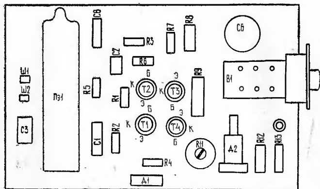
Рис. 13. Расположение элементов на плате калибратора
