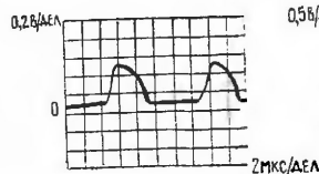
Рис. 20. База транзистора T31
