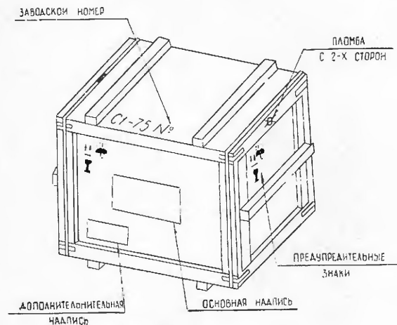
Рис. 26. Схема маркировки:
