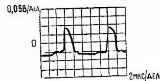
Рис. 22. База транзистора T26
