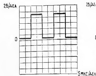
Рис. 23. Коллектор транзистора Т1
