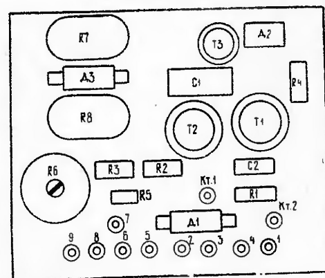
Рис. 18. Расположение элементов на плате мостов
