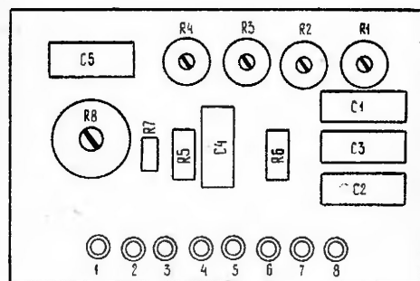
Рис. 14. Расположение элементов на плате управления режимом ЭЛТ
