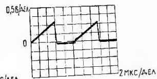
Рис. 15. Коллектор транзистора T24
