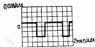
Рис. 19. База транзистора T13
