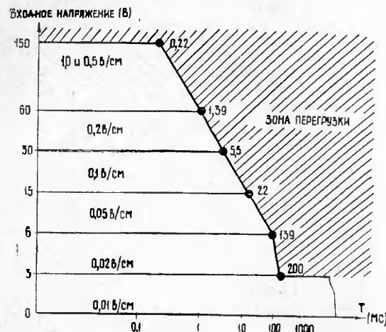
Рис. 14. Зависимость величины импульсного входного напряжения от длительности импульса T для однократных сигналов
