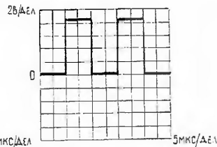
Рис. 26. Эмиттер транзистора Т4
