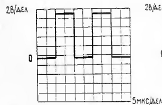
Рис. 25. Коллектор транзистора Т3
