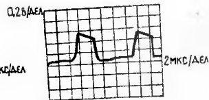
Рис. 18. База транзистора T15
