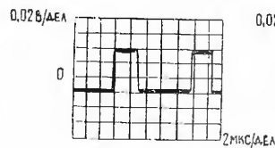
Рис. 9. Коллектор транзистора Т8
