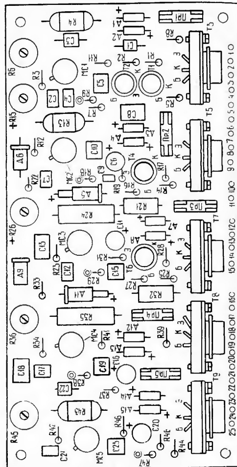
Рис. 15. Расположение элементов на плате стабилизаторов
