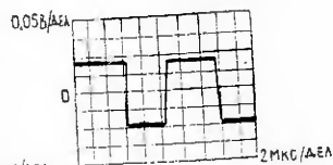
Рис. 13. База транзистора T22
