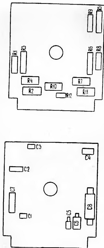
Рис. 7. Расположение элементов на плате переключателя развертки
