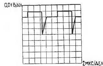
Рис. 30. Точка 2 на плате
