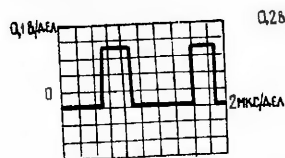
Рис. 17. Коллектор транзистора T14
