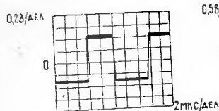
Рис. 14. Коллектор транзистора T22
