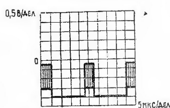
Рис. 1. Контакт 6 микросхемы МС2
