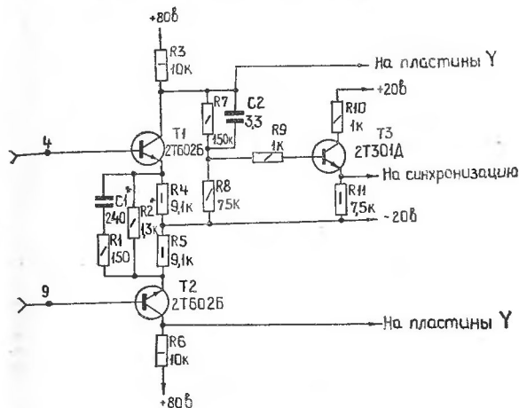
Рис. 5. Оконечный каскад.
