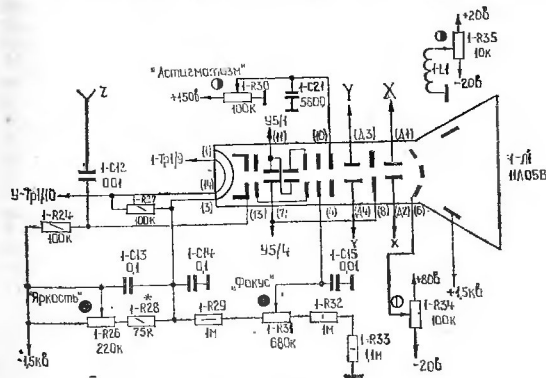
Рис. 14. Индикатор (ЭЛТ).
