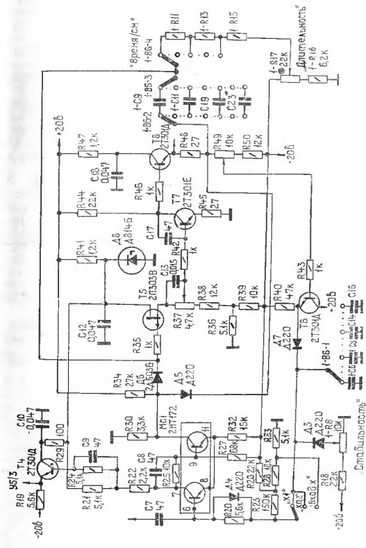
Рис. 8. Схема развертки.
