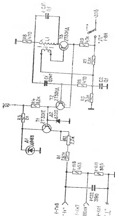
Рис. 6. Калибратор
