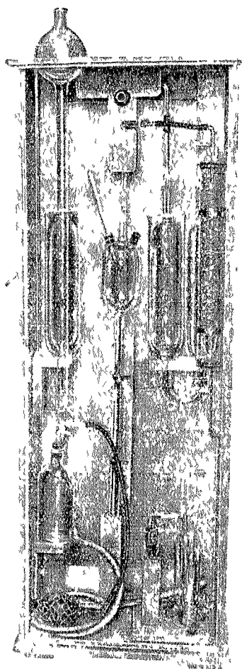
Газоанализатор типа ГОУ
