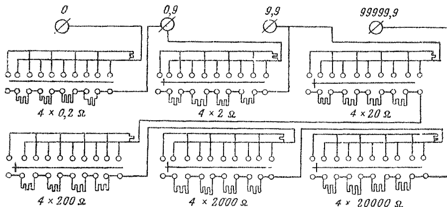
Схема магазина сопротивлений типа КМС-6
