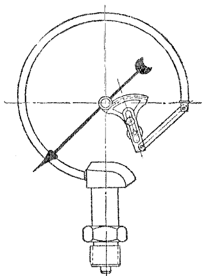
Схема манометра
