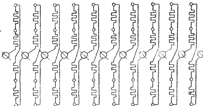
Схема магазина сопротивлений типа МСВ
