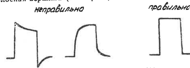
Черт. 7. Осциллограммы импульсов.
