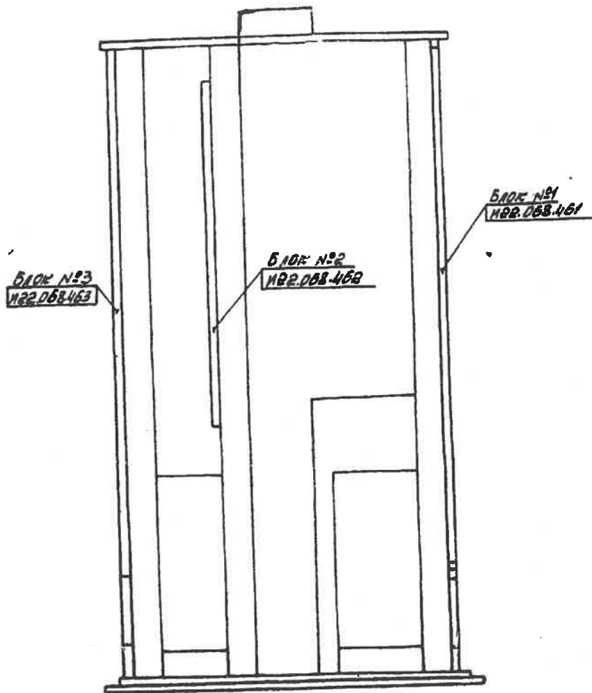
Черт. 4. Схема расположения установочных элементов блока БВС (вид сверху)
