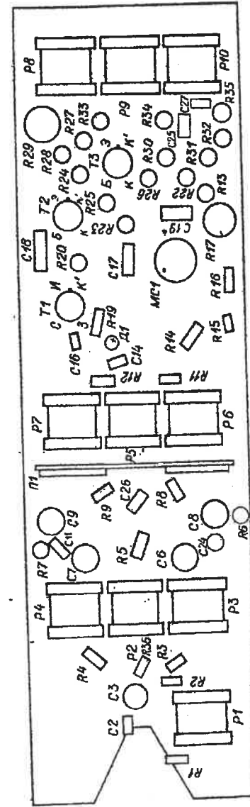
Аттенуатор. Схема расположения ЭРЭ
