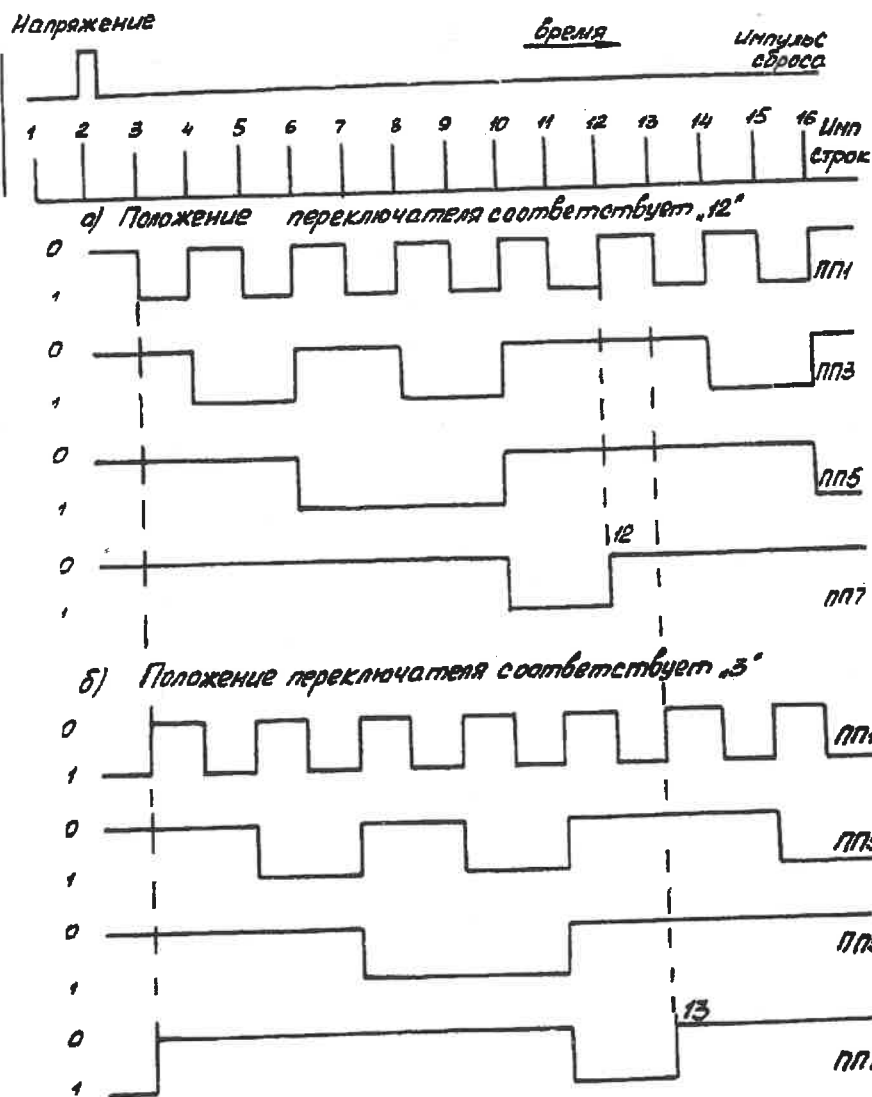
Черт. 3. Временные диаграммы
