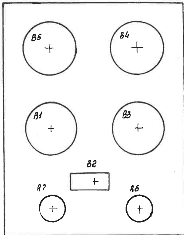
Черт. 6. Передняя панель блока БВС (вид с внутренней стороны)
