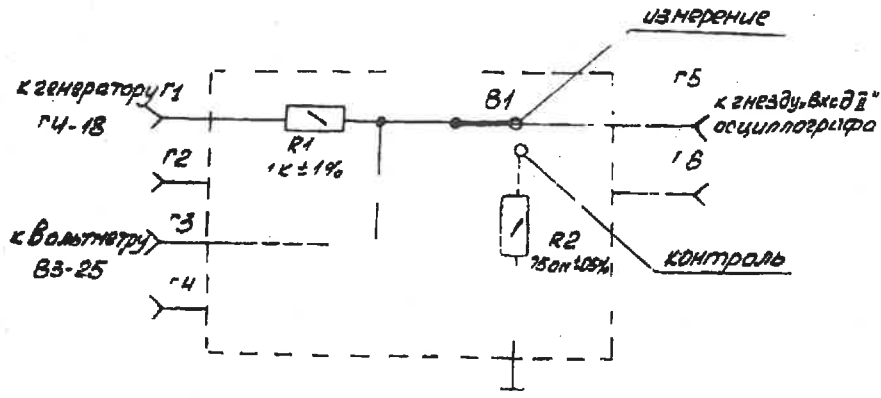
Схема измерительной приставки
