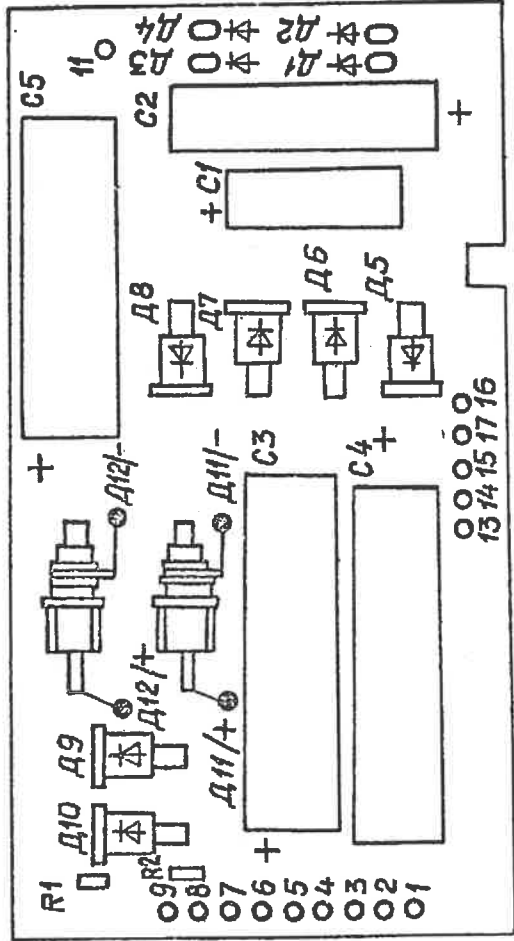
Блок питания (У1) . Плата П2. Схема расположения ЭРЭ
