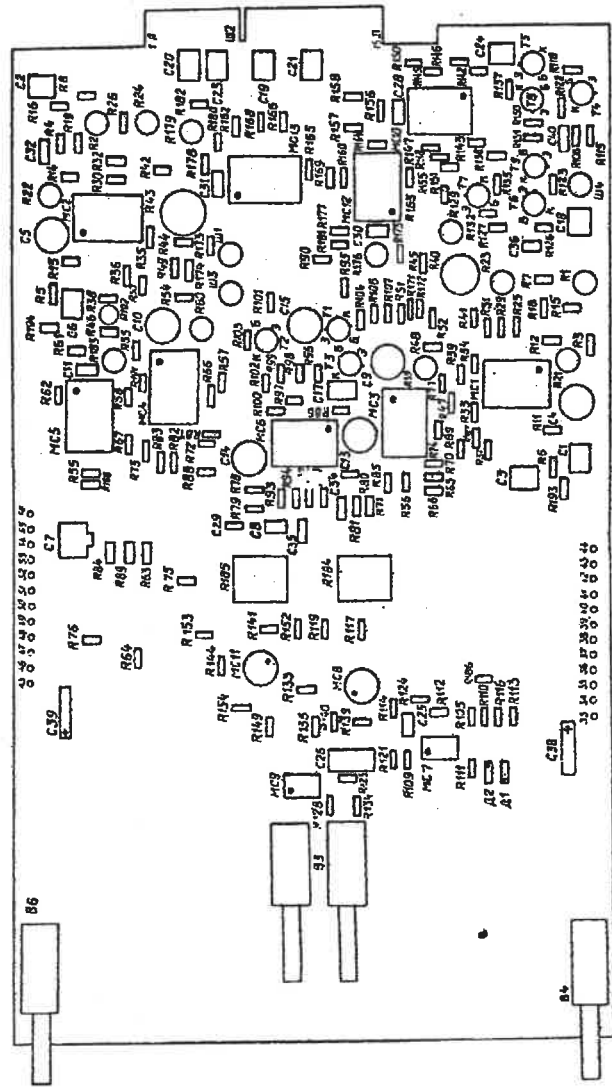
Усилитель вертикального отклонения Схема расположения ЭРЭ
