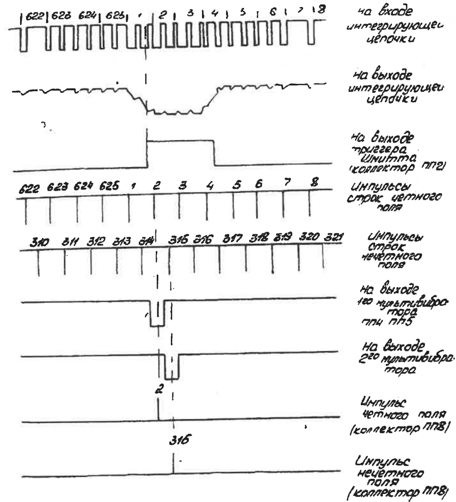
Черт. 2. Временные диаграммы.
