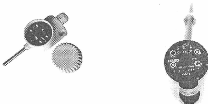
Рис.3 - Общий вид термопреобразователей сопротивления со встроенным нормирующим преобразователем
