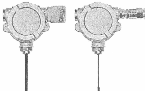
Рис.8 Взрывозащищенные ТСп-Exd, ТСп-Exdi для измерения температуры окружающей среды (воздуха)
