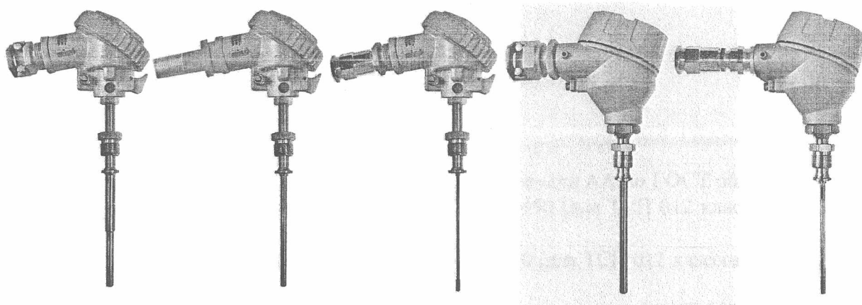
Рис.5 Погружаемые взрывозащищенные ТС-Ехd, ТС-Ехd i
