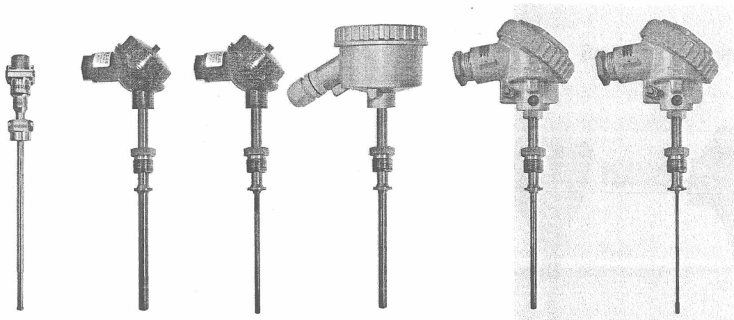
Рис.1 Погружаемые общепромышленные ТС-Оп и взрывозащищенные ТС-Ехi
