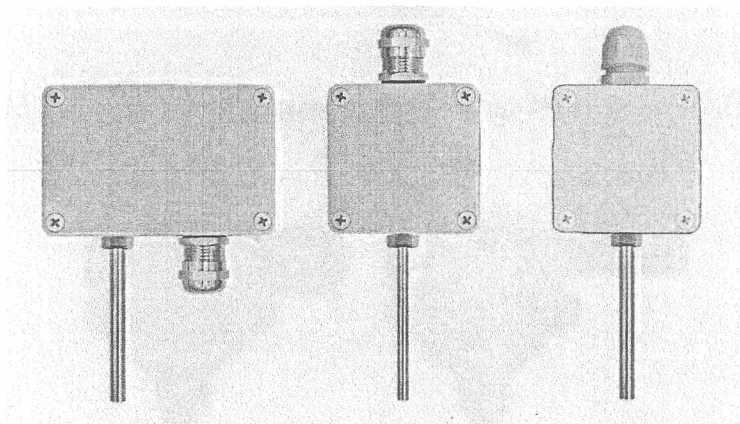
Рис.4 Общепромышленные ТСп-Оп и взрывозащищенные ТСп-Ехi для измерения температуры окружающей среды (воздуха)
