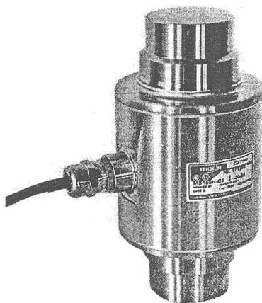
Рисунок 1 – Внешний вид датчиков МВ 150.
