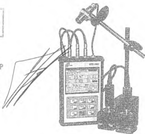
Рисунок 1 - Виброанализатор STD-3300
