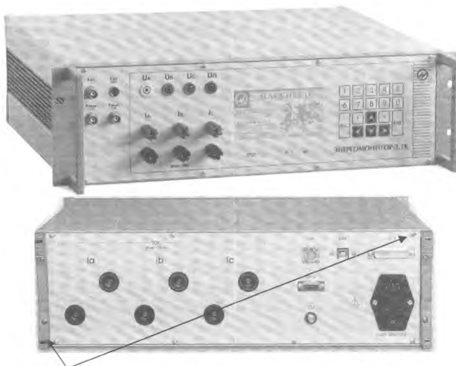
Рисунок 2. Общий вид и места пломбировки Приборов модификаций "Энергомонитор-3.1К М" Н
