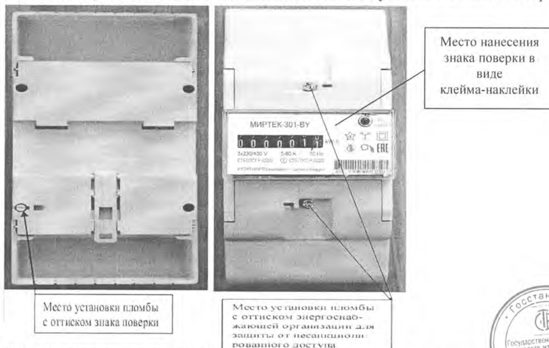
Рисунок А.5 – Места установки пломб и нанесения знака поверки для счетчиков в корпусе модификации D34
