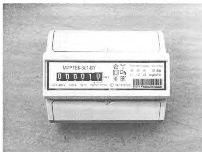
Рисунок 8 – Общий вид счетчика в корпусе модификации D36
