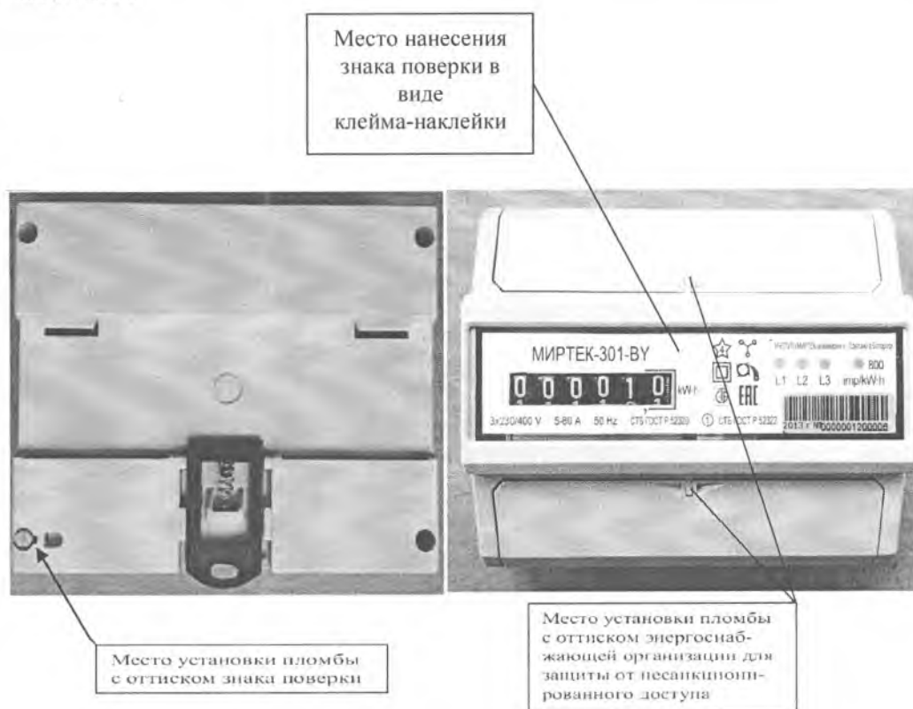
Рисунок А.6 – Места установки пломб и нанесения знака поверки для счетчиков в корпусе модификации D35
