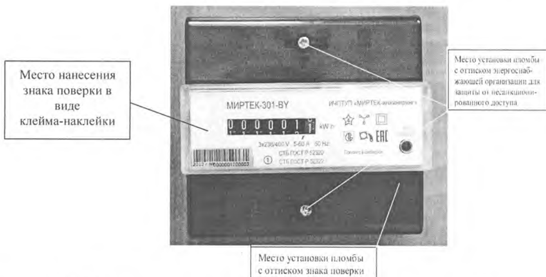
Рисунок А.3 – Места установки пломб и нанесения знака поверки для счетчиков в корпусе модификации D32
