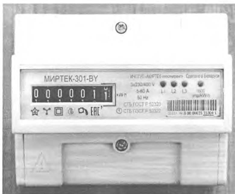
Рисунок 5 – Общий вид счетчика в корпусе модификации D33
