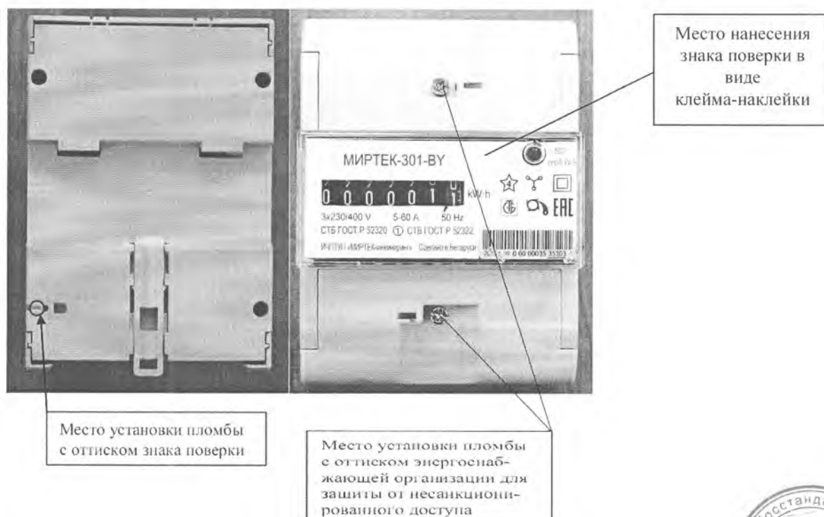
Рисунок А.2 – Места установки пломб и нанесения знака поверки для счетчиков в корпусе модификации D31
