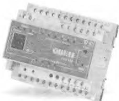
Рис.1 - Общий вид контроллеров логических программируемых ОВЕН ПЛК150
