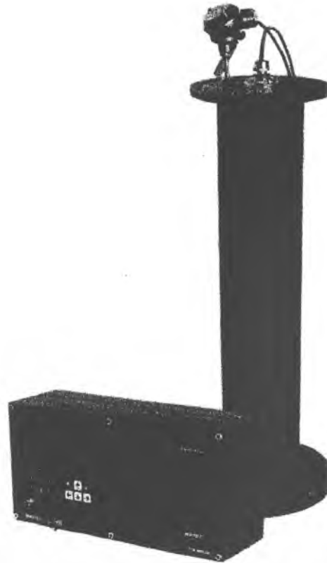
Рисунок 1 - Общий вид расходомеров-счетчиков ультразвуковых «ВЗЛЕТ РСЛ»
