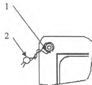
Рисунок. 2 - Схема пломбировки расходомеров-счетчиков ультразвуковых «ВЗЛЕТ РСЛ»
