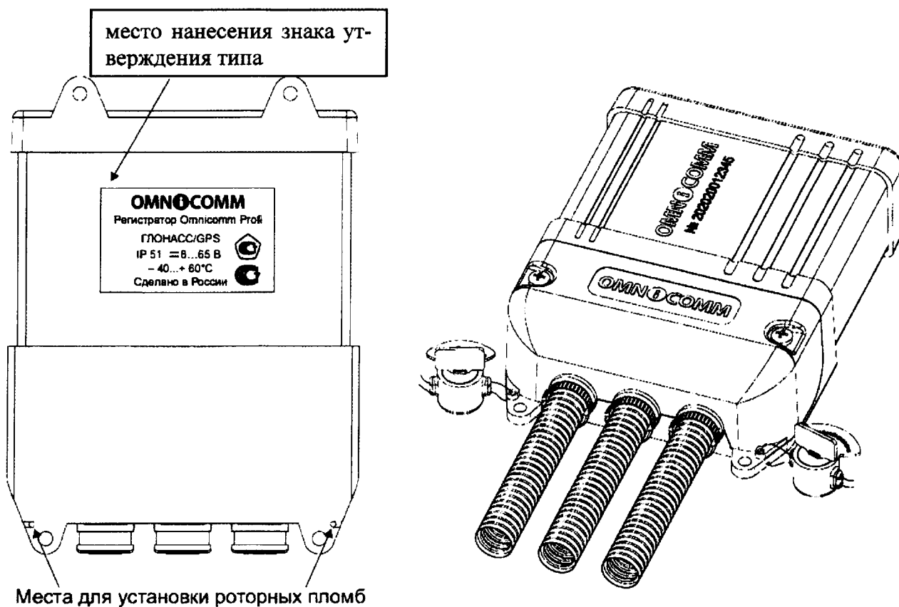
Рисунок 1 - Внешний вид аппаратуры Omnicomm Profi
