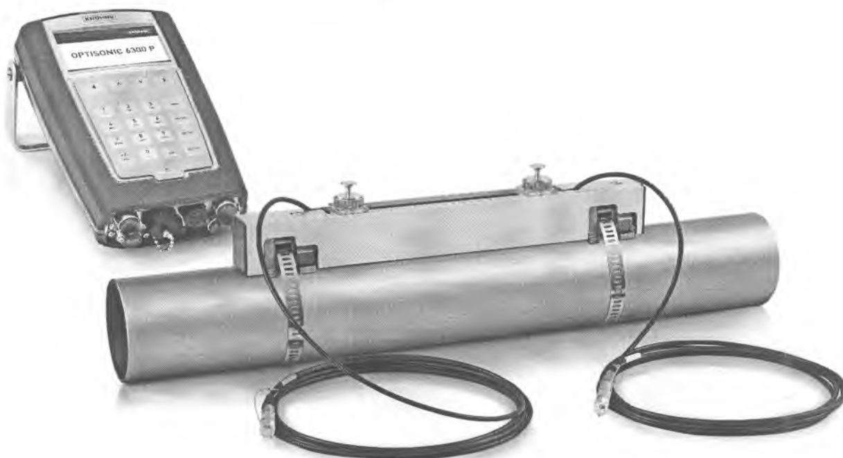
Рис.1 Общий вид расходомера ультразвукового портативного с накладными датчиками OPTISONIC 6300 P
