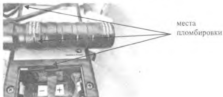
Рисунок 2 - Схема пломбировки твердомера.
