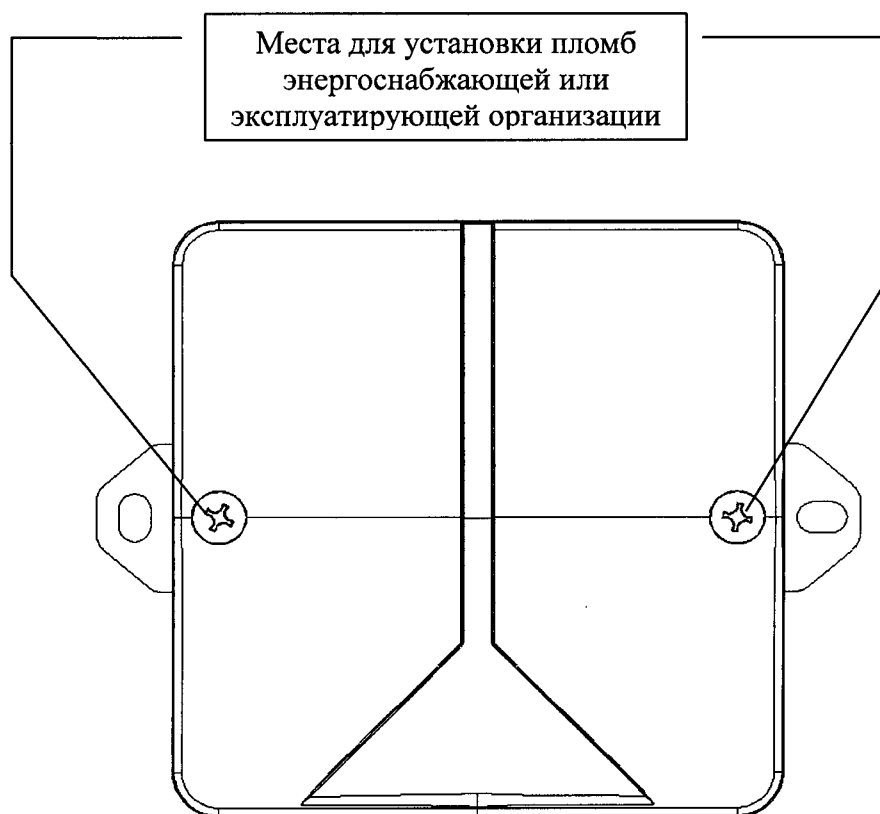
Рисунок А.3 – Схема пломбировки сумматора CE826-02
