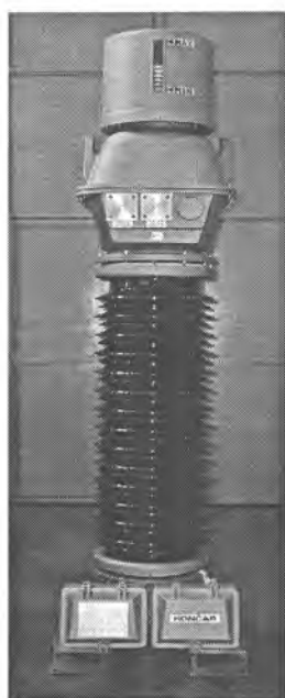
Рисунок 1 Внешний вид трансформаторов VAU-123, VAU -245, VAU -362.
