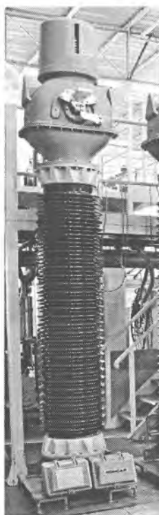
Рисунок 1 Внешний вид трансформаторов VAU-123, VAU -245, VAU -362.
