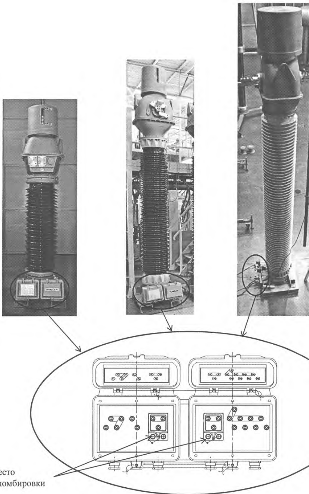
Рисунок 2 Схема пломбировки трансформаторов VAU-123, VAU -245, VAU -362.
