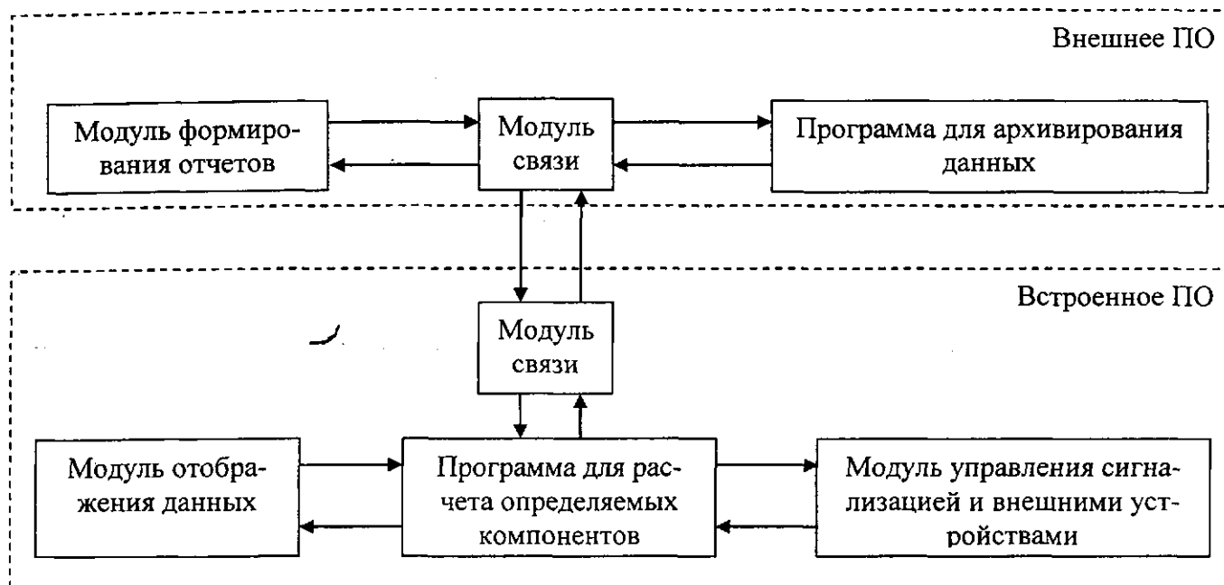
Рисунок 1 - Структура ПО.
