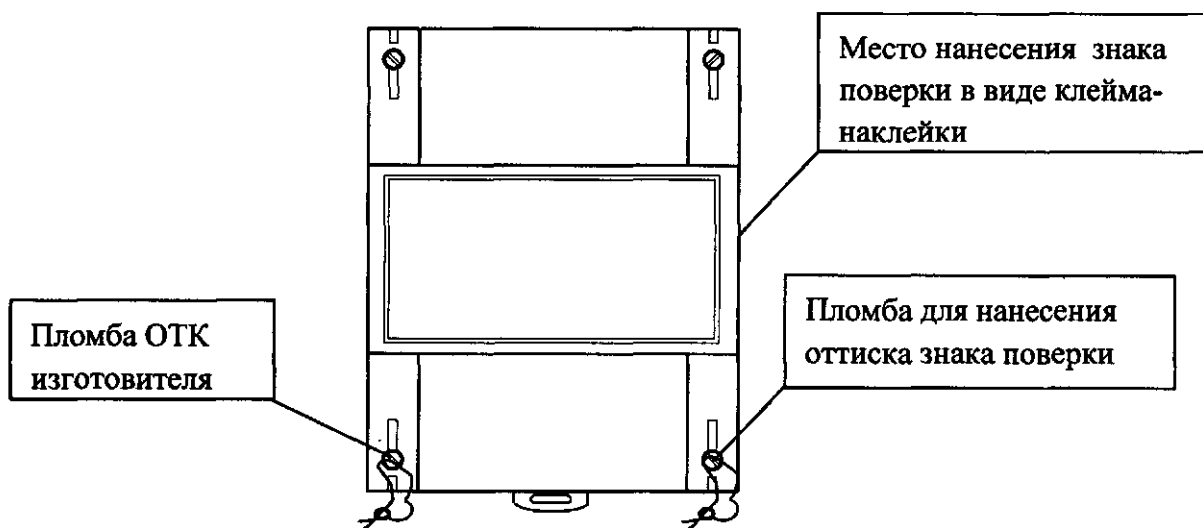
Рисунок А – Корпус УСПД 164-01Б-0 и УСПД 164-01Б-1
