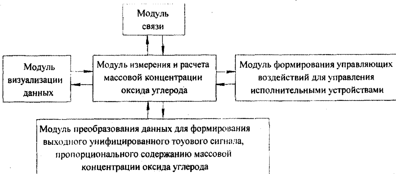
Рисунок 3 - Структура ПО
