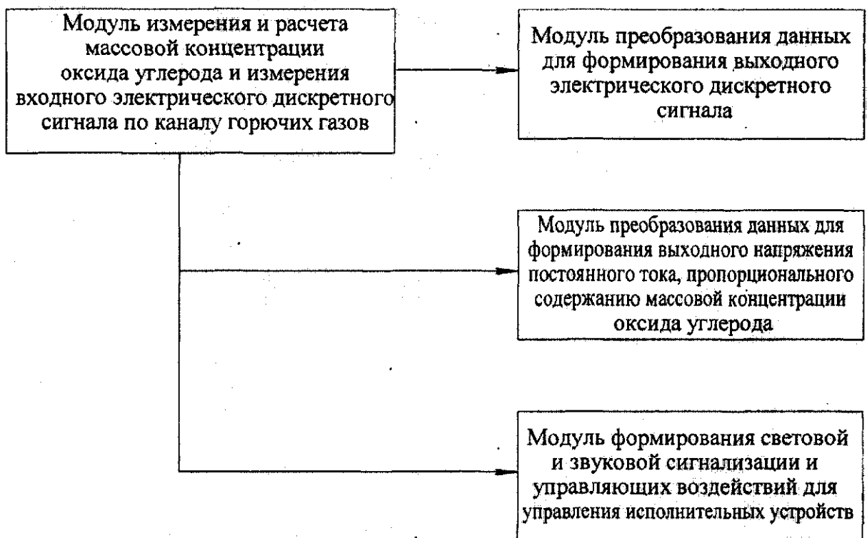
Рисунок 3 - Структура ПО.
