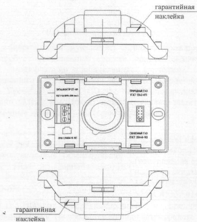
Рисунок 2 - Схема пломбировки сигнализаторов от несанкционированного доступа и обозначение мест для нанесения гарантийных наклеек
