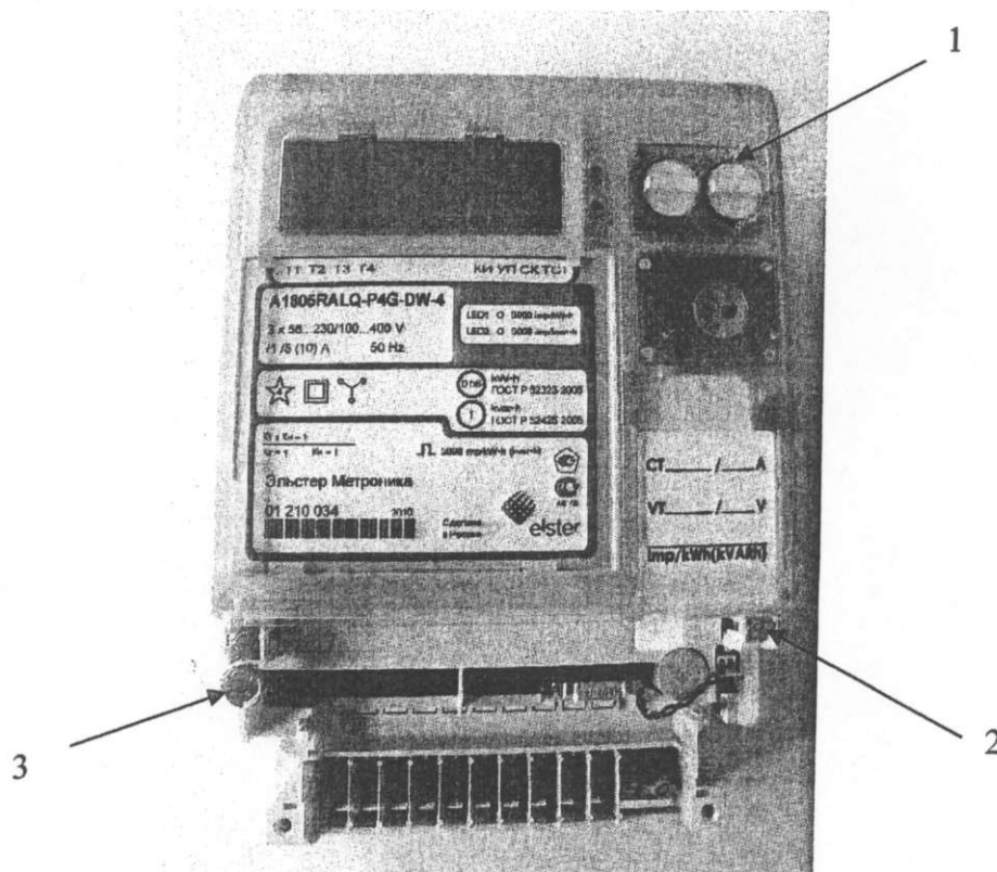
1 - пломба кнопки СБРОС; 2 - пломба поверителя; 3 - пломба ОТК завода-изготовителя
