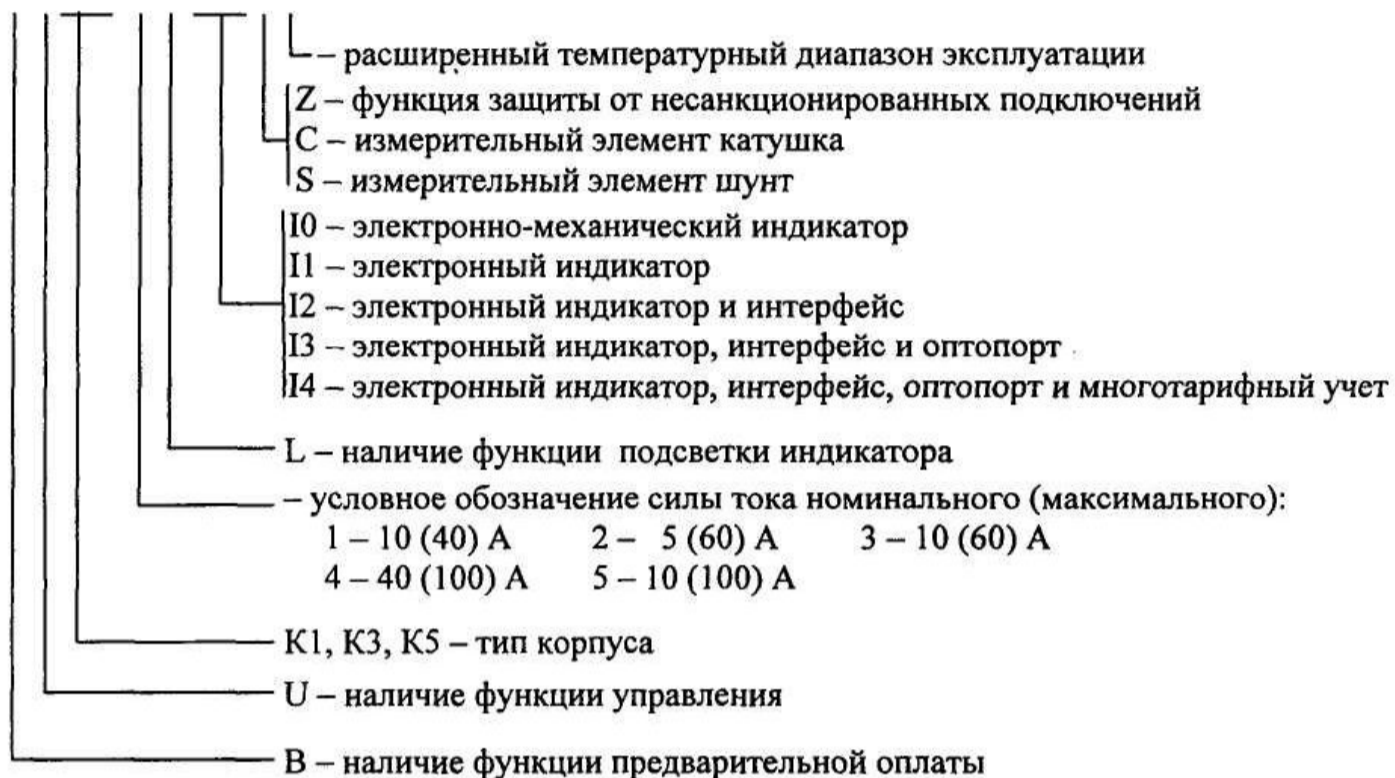
Рисунок 1 – Схема построения обозначения возможных исполнений однофазного счетчика «Энергия - 9»
