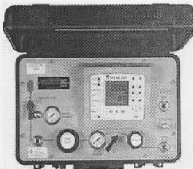
Рисунок 5. Внешний вид калибраторов DPI 320.
