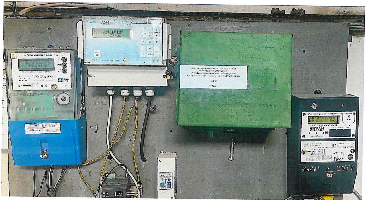
а) сумматор и счётчики из состава АСКУЭ
