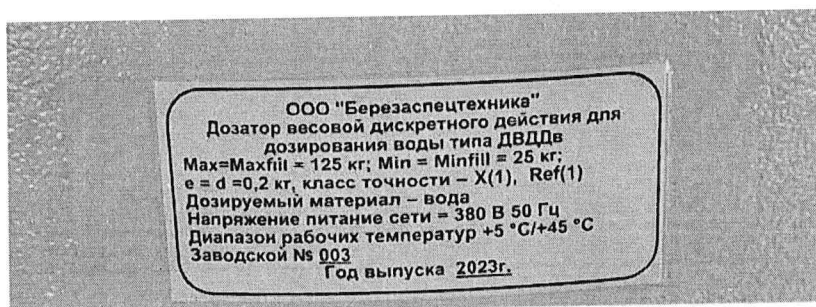
Рисунок 1.2 – Фотография маркировки дозатора весового дискретного действия для дозирования воды типа ДВДв № 003
