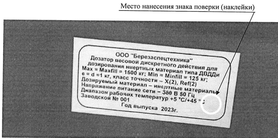
Рисунок 2.1 - Фотография с указанием места нанесения знака поверки (наклейки) на маркировочную табличку дозатора весового дискретного действия для дозирования инертных материалов типа ДВДДи № 001
