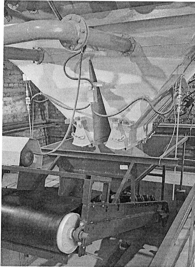
Рисунок 1.1 – Фотография внешнего вида дозатора весового дискретного действия для дозирования инертных материалов типа ДВДДи № 001
