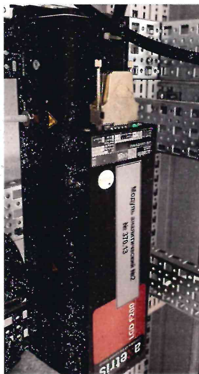
Рисунок 1.6 – Фотография общего вида модуля лазерного LGD LGD F200P2-H NH 3
