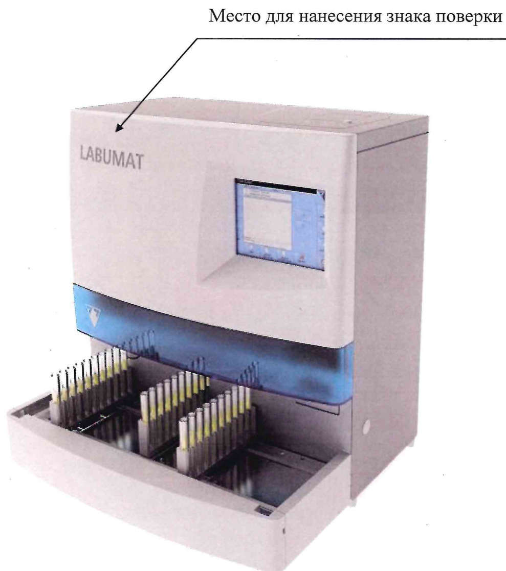
Рисунок 2.1 – Схема с указанием места для нанесения знака поверки на анализатор мочи LabUMat 2 № UPA08000172
