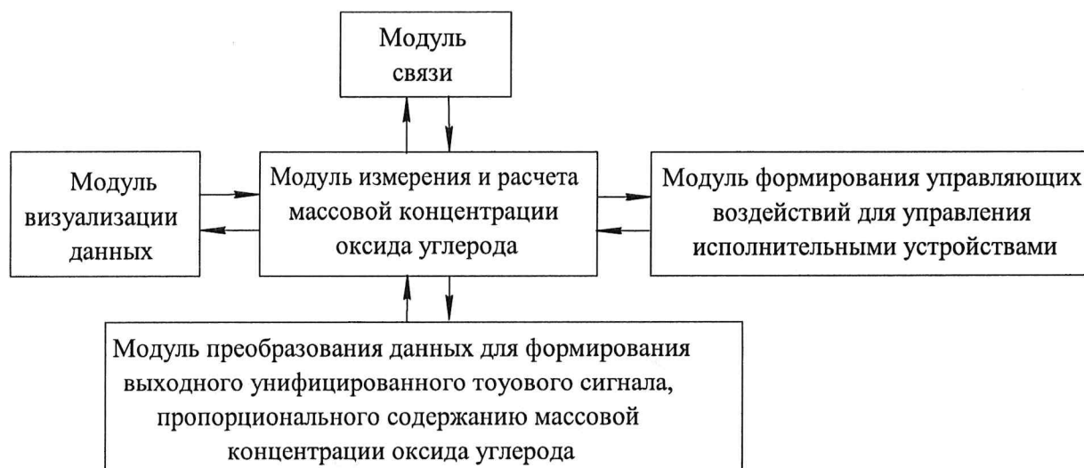
Рисунок 3 - Структура ПО
