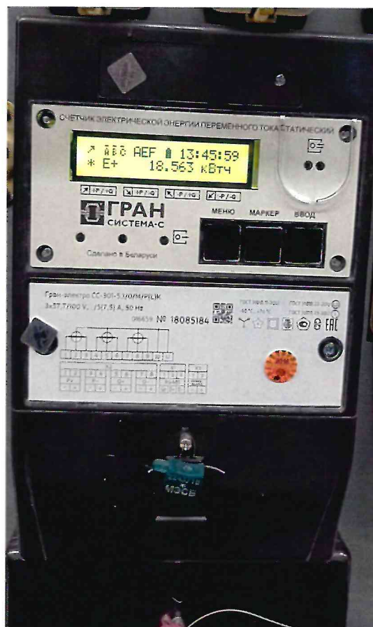
Рисунок 1.2 – Фотографии счётчиков, входящих в состав измерительных каналов АСКУЭ (изображение носит иллюстративный характер)
