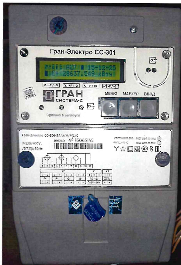
Рисунок 1.2 – Фотографии счётчиков, входящих в состав измерительных каналов АСКУЭ (изображение носит иллюстративный характер)
