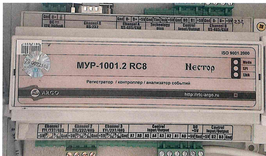
б) КИИ «МУР 1001» в шкафу АСКУЭ
