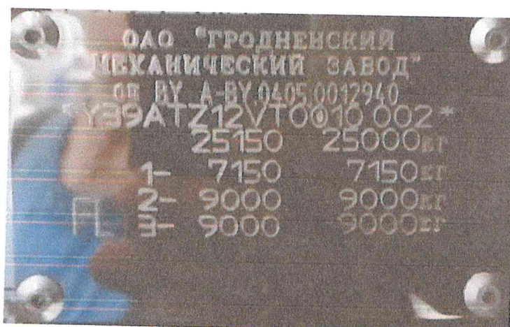
Рис.3 Табличка изготовителя в кабине водителя
