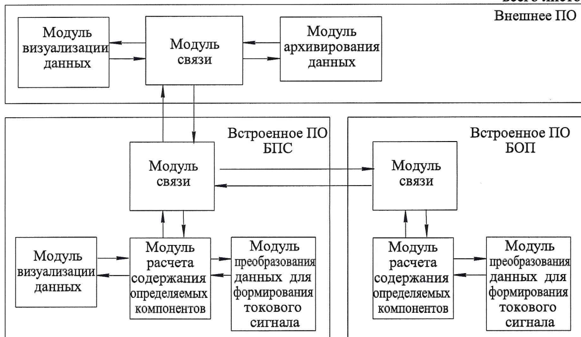
Рисунок 1 - Структура ПО
