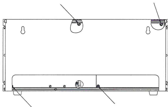
Рисунок 3 - Схема пломбировки газоанализаторов от несанкционированного доступа и обозначение мест для нанесения оттисков клеем
