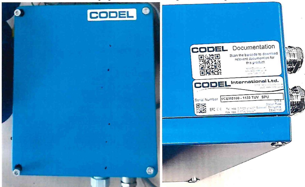
Рисунок 1.4 – Фотография маркировки сигнального процессора. Измеритель скорости газовоздушных потоков VCEM5100 № VCEM5100 – 1133 TUV SPU
