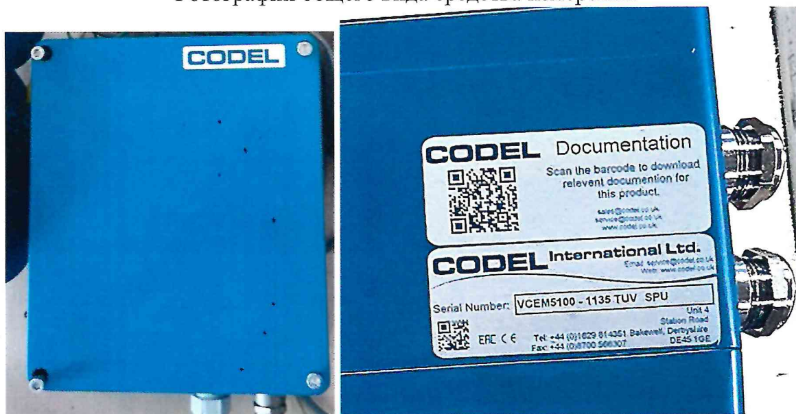
Рисунок 1.4 – Фотография маркировки сигнального процессора. Измеритель скорости газовоздушных потоков VCEM5100 № VCEM5100 – 1135 TUV SPU
