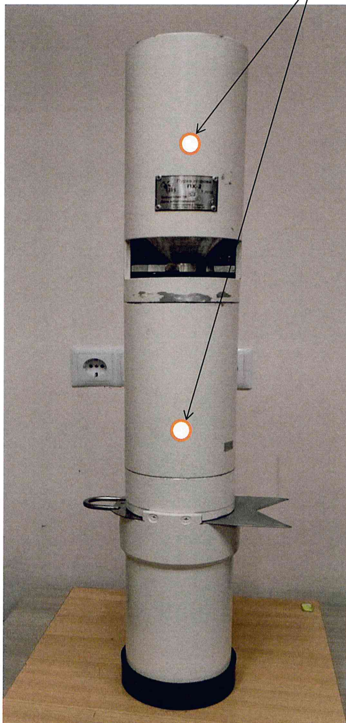
Рисунок 2.1 - Фотография с указанием места нанесения знака поверки (наклейки) на пурку литровую рабочую с падающим грузом ПХ-2 № 1530
