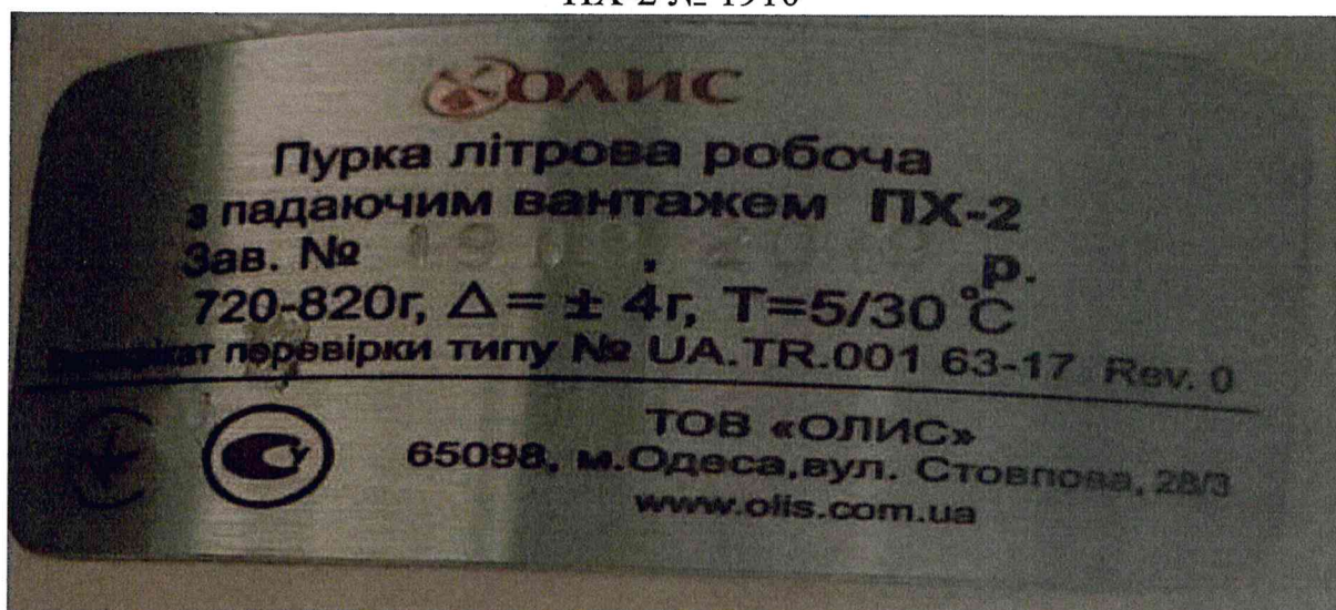
Рисунок 1.1 - Внешний вид пурки литровой рабочей с падающим грузом ПХ-2 № 1910
